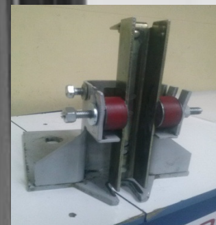
AMORTIGUADORES EN POLIURETANO
